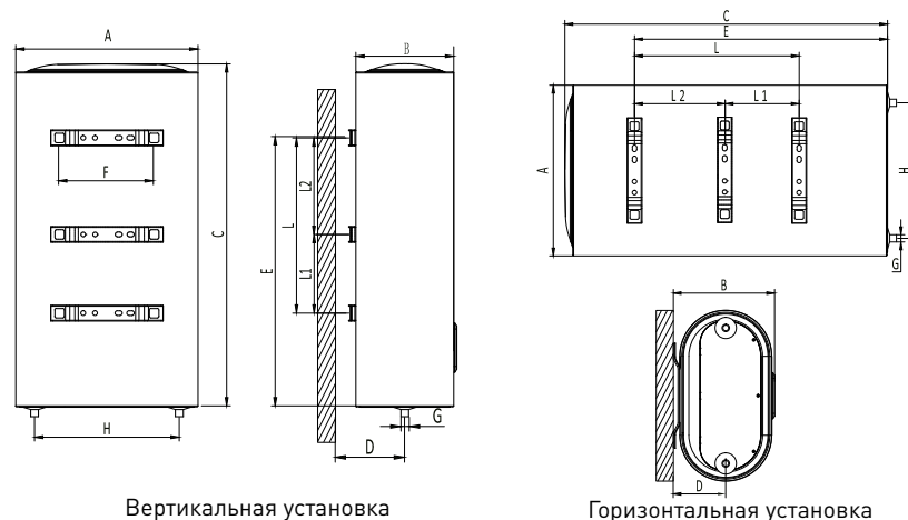
Вертикальная установка
