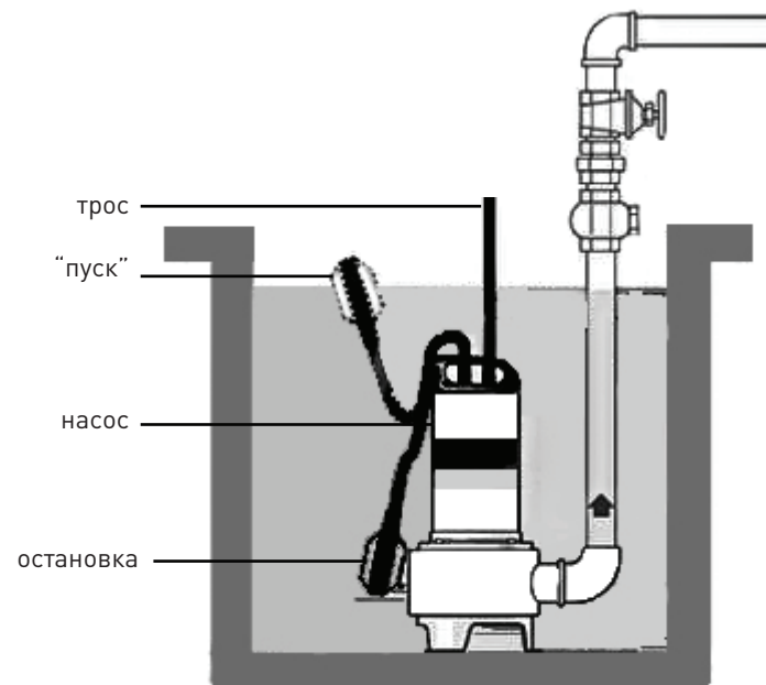
Схема погружения насоса
