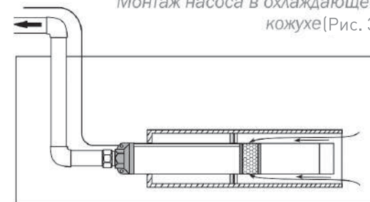
Монтаж насоса в охлаждающем
