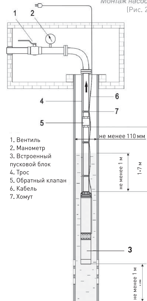
Монтаж насоса в охлаждающем
