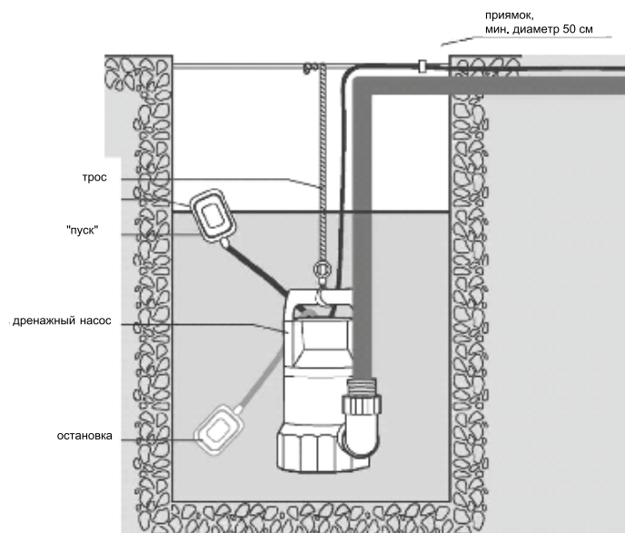
Схема погружения насоса
