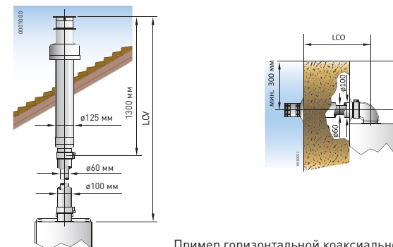
Пример горизонтальной коаксиальной системы (C12)
