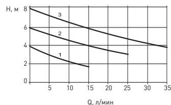
Рабочее поле для насоса CV - 25/8
