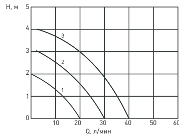
Рабочее поле для насоса CV - 25/4
