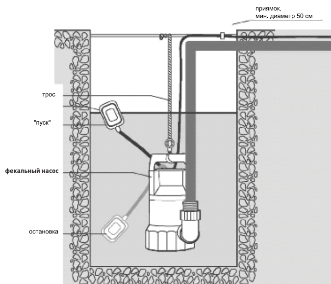
Схема погружения насоса
