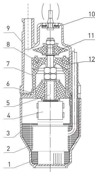
Рис. 1. Устройство насоса
